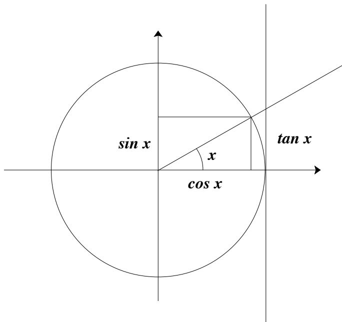
FIGURE 1.1 – Représentation géométrique des grandeurs \cos x , \sin x et \tan x .
