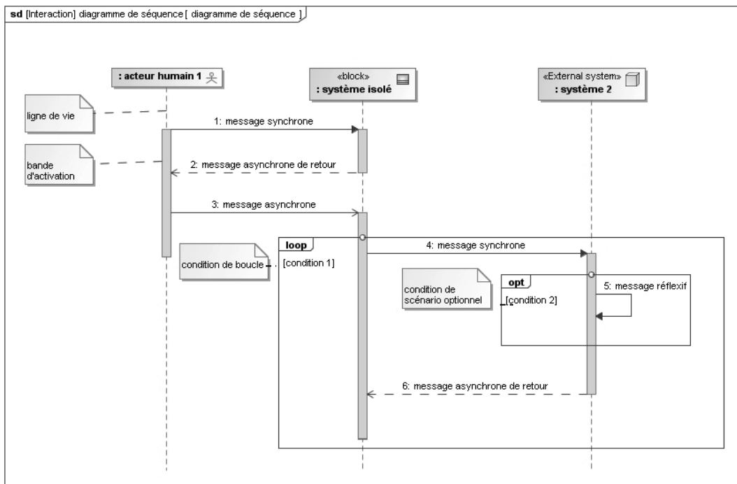
⇒ Méthode 1.4. Lecture et construction d'un diagramme de séquence
